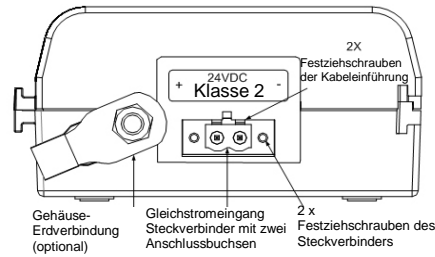
Abbildung 2: PoE Midspan Leistungssteckverbinder
