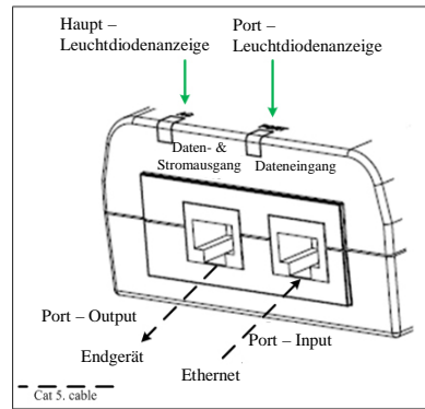
Abbildung 3: PoE Midspan Ports
