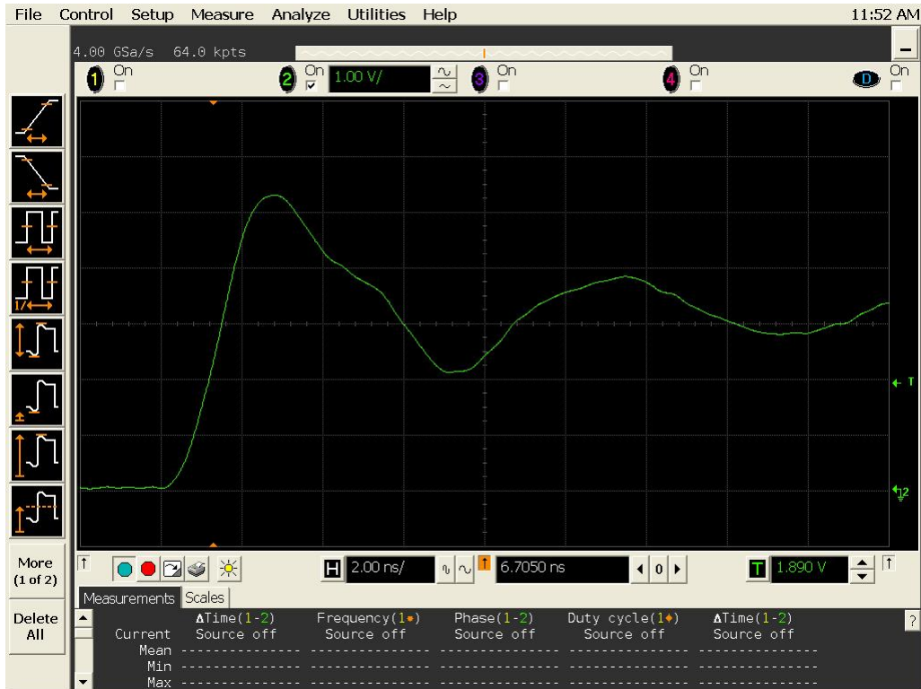
Figure 12b DUT 16373 Post-Annealing Rising Edge
