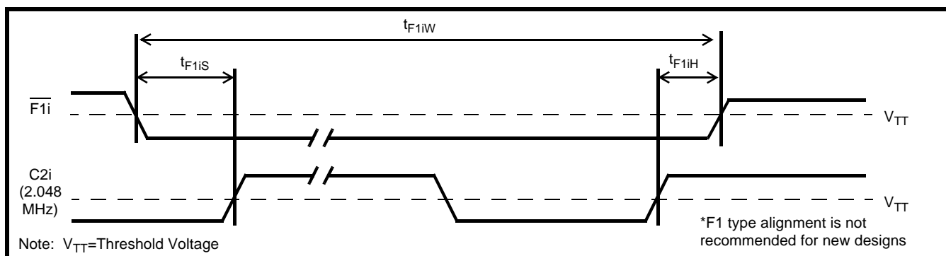
Figure 4 - F1 Type Frame Pulse
